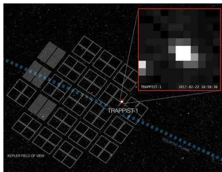
Fig. 2 Prawdziwy obraz układu TRAPPIST-1 widziany przez teleskop
