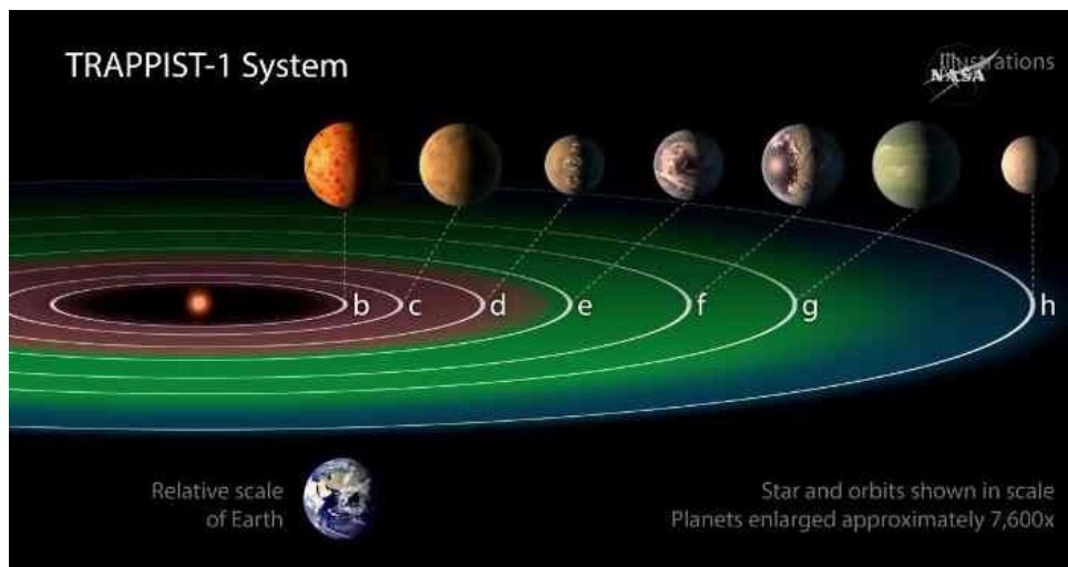
Fig. 1 Wizja układu TRAPPIST-1 przygotowana przez naukowców
